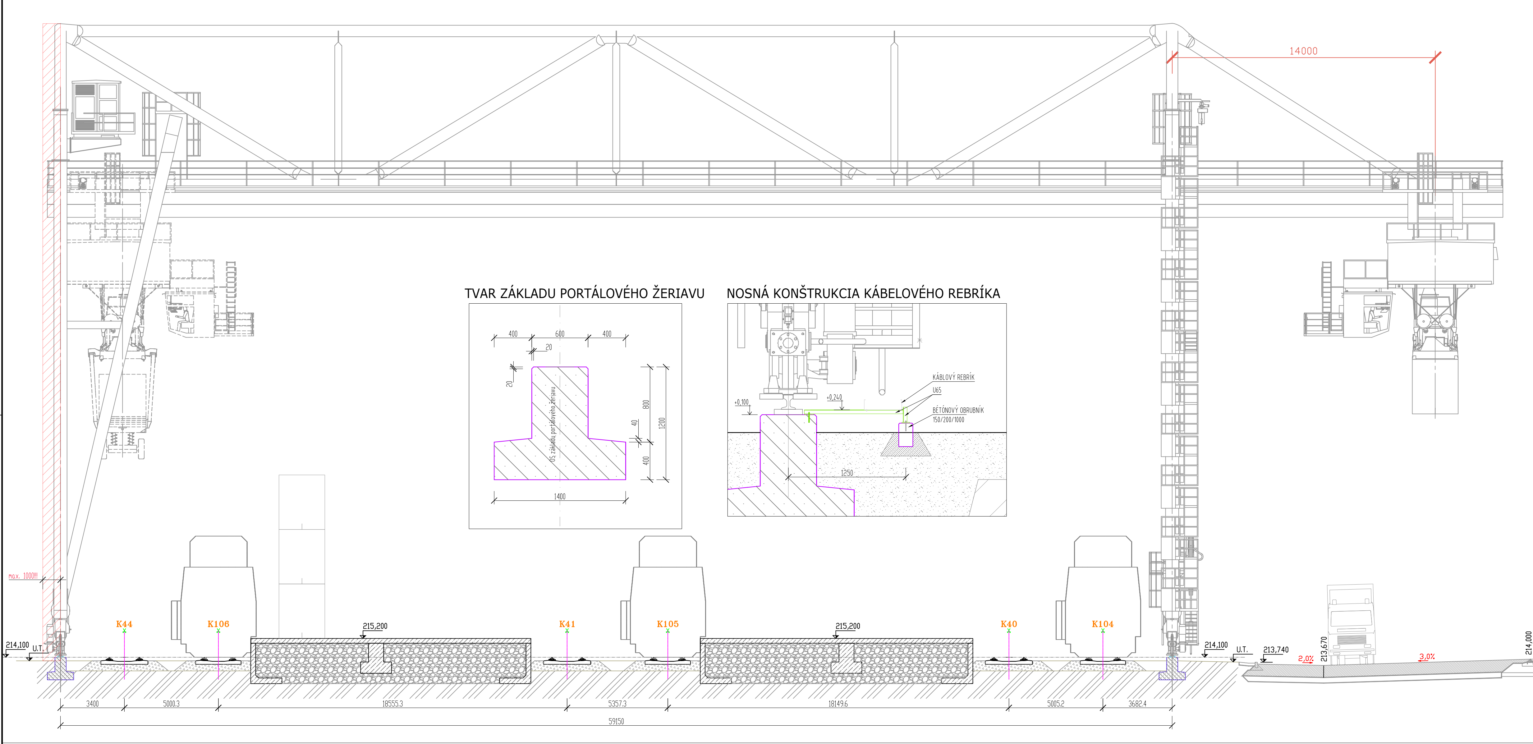
SCHÉMATICKÝ REZ PORTÁLOVÝM ŽERIAVOM
