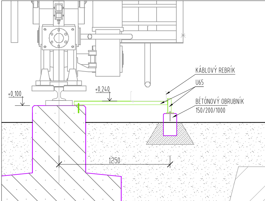
NOSNÁ KONŠTRUKCIA KÁBELOVÉHO REBRÍKA
