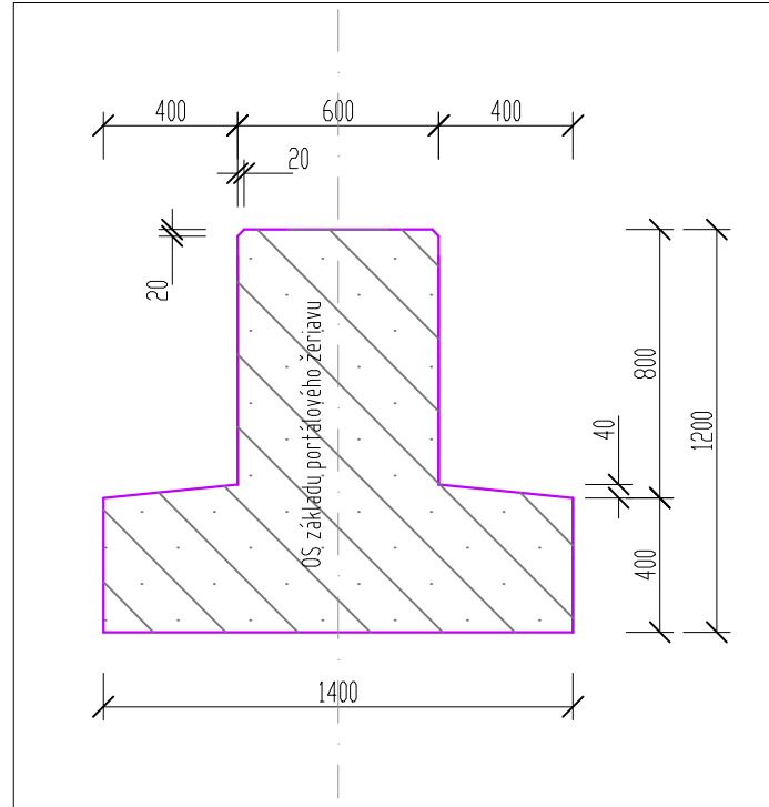
TVAR ZÁKLADU PORTÁLOVÉHO ŽERIAVU
