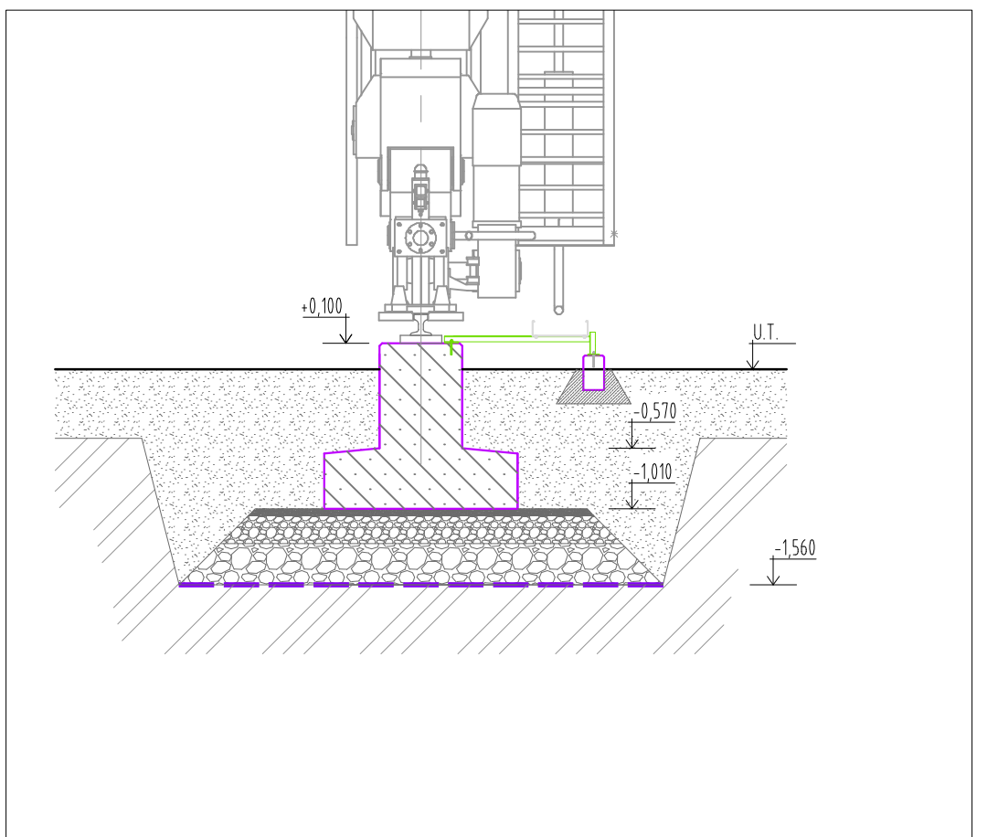
SCHÉMATICKÝ REZ ZÁKLADOM PORTÁLOVÉHO ŽERIAVU
