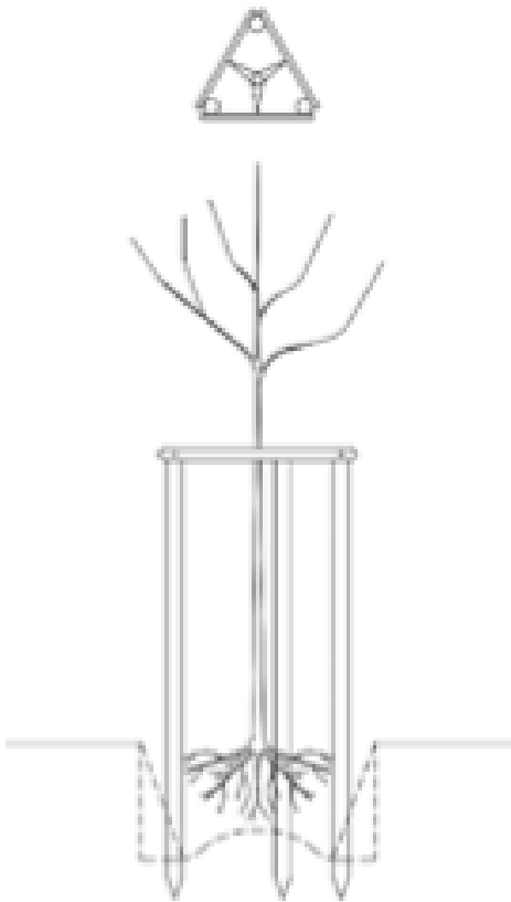
Obr. 1 - Nadzemné kotvenie stromov
