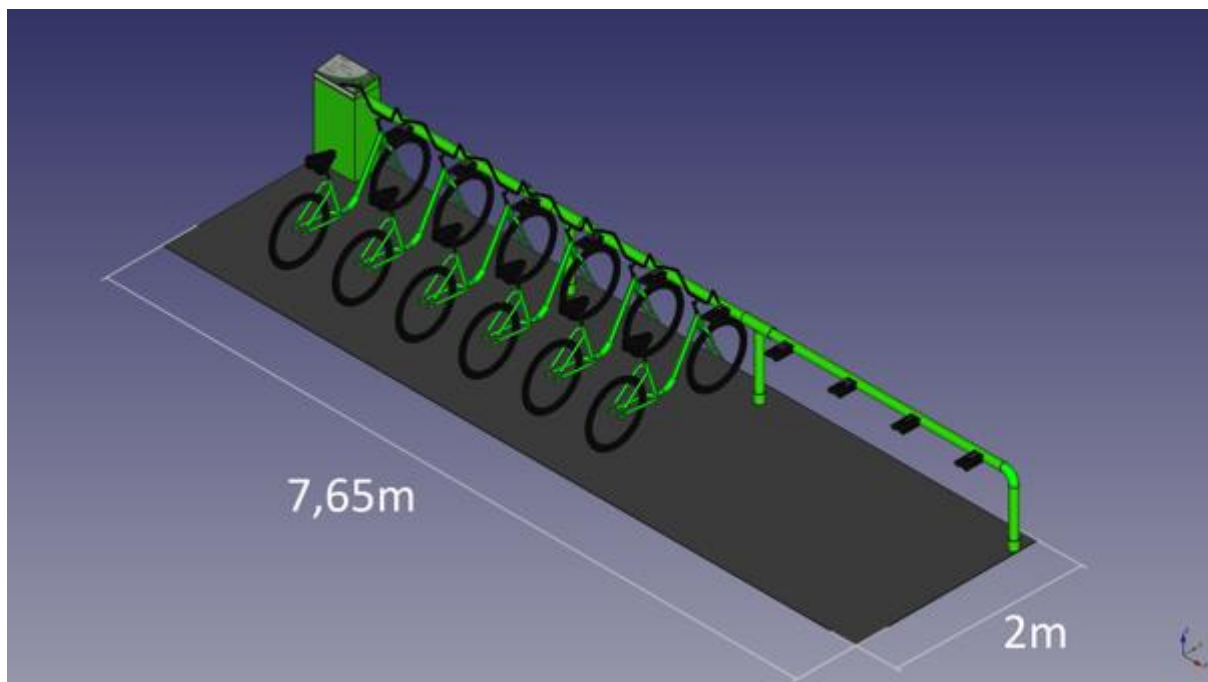
Nákres stojanu pre s desiatimi parkovacími miestami
