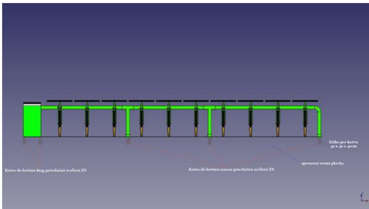
Pohľad zpredu na stojan s desiatimi parkovacími miestami so spôsobom ukotvenia
