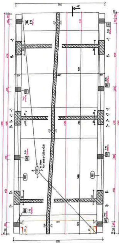
TVAR STROPNEJ DOSKY 41220
