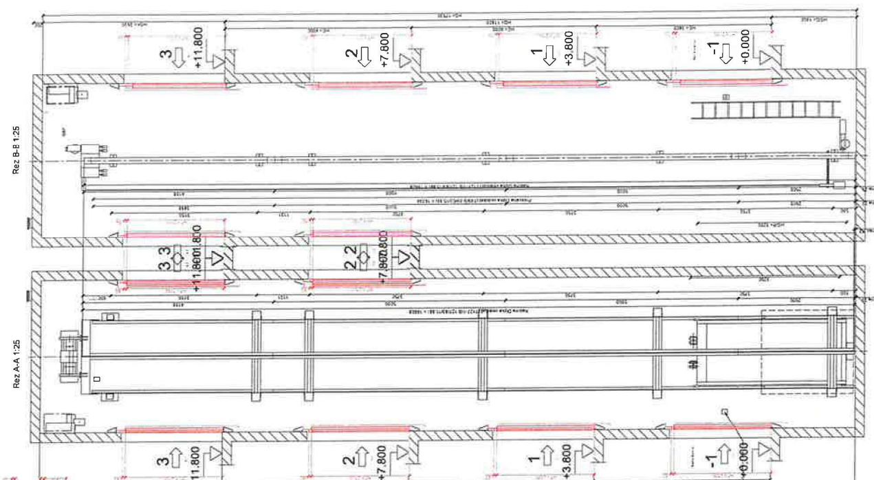
Priehľad šachty 120
