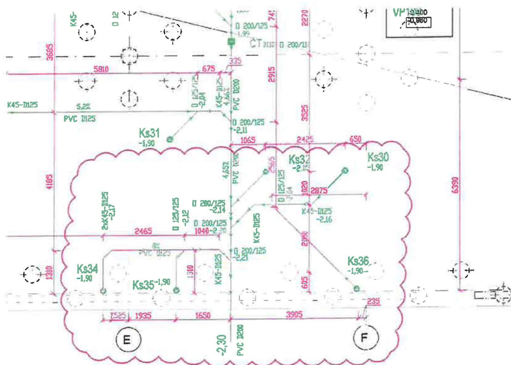
Úpravu trasovania splaškovej kanalizácie pre stúpačky Ks34 a Ks36 (SO 02) (Printscreen z prílohy č.1)
