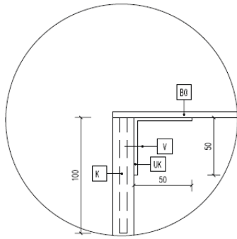
DET. 1 UHOLNÍKOVÉ KOTVENÍ - PRIVARENÉ K PLECHU, DO DŘEVA VRUT
