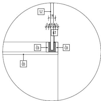
DET. 3 DRÁŽKA S GUMOVÝM TESNENÍM NA KOTVENIE SKLENÉHO ŽÁKLUPU
