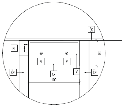
DET. 1 KOTVIACI PRVKOV - PRIVARENÉ K PLECHU, DO DŘEVA VRUT
