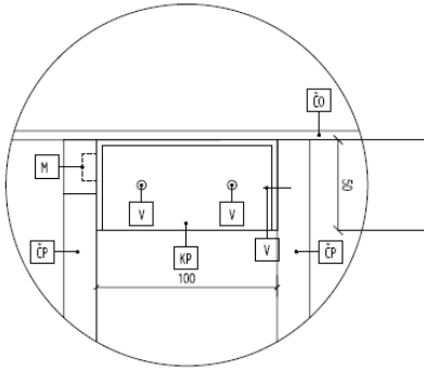
DET. 1 KOTVIACI PRVOK - PRIVARENÉ K PLECHU, DO DŘEVA VRUT
