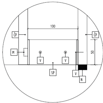
DET. 2 KOTVIACI PRVKOV - PRIVARENÉ K PLECHU, DO DŘEVA VRUT
