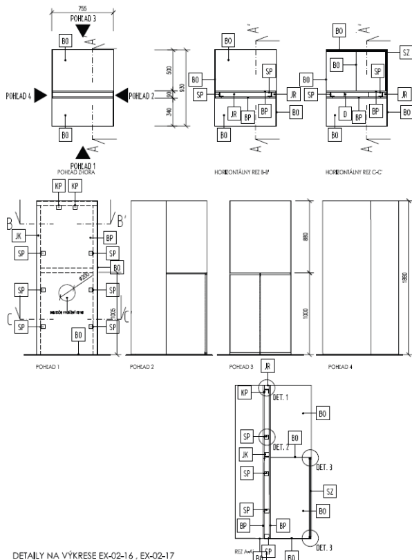
DETAILY NA VÝKRESĚ EX-02-16, EX-02-17
