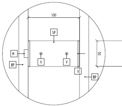
DET. 2 SPOJOVACÍ PRVOK - PRIVARENÉ K PLECHU, DO DREVA VRUT
