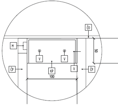
DET. 1 KOTVIACI PRVKOK - PRIVARENÉ K PLECHU, DO DREVA VRUT
