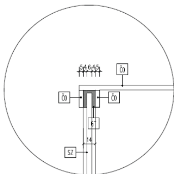
DET.3 DRÁŽKA S GUMOVÝM TESNENÍM NA KOTVENIE SKLENÉHO ZÁKLAPU
