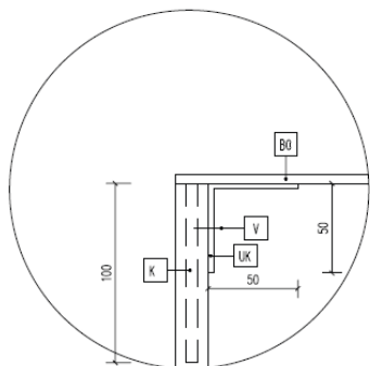
DET. 1 UHOLNÍKOVÉ KOTVENIE - PRIVARENÉ K PLECHU, DO DŘEVA VRUT
