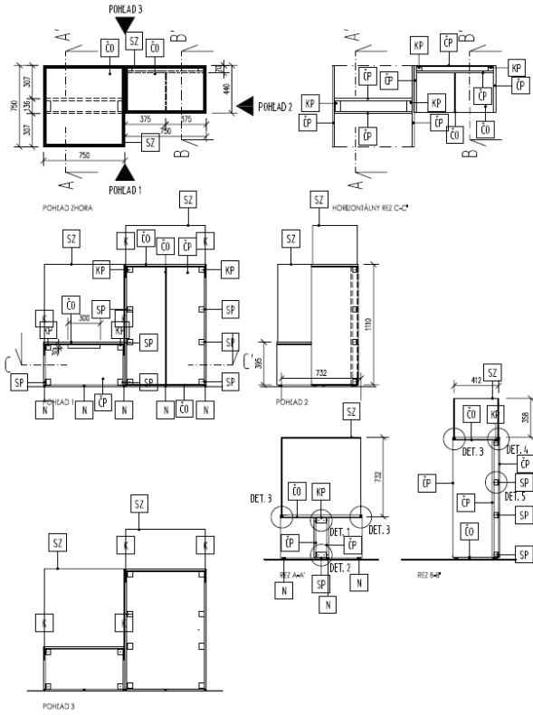
DETAILY NA VÝKRESE EX-02-41, EX-02-42, EX-02-43
