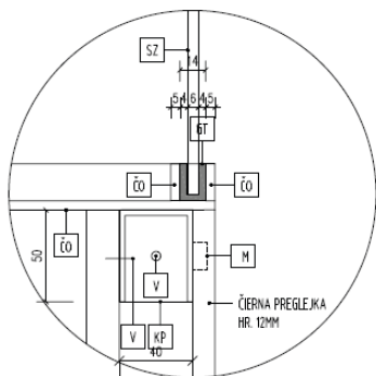
DET. 4 KOTVIACI PRVK - PRIVARENÉ K PLECHU, DO DREVA VRUT
