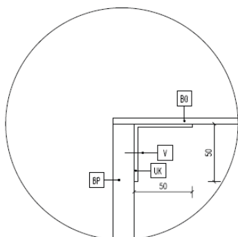
DET.1 UHOLNÍKOVÉ KOTVENIE - PRÍVARENÉ K PLECHU, DO DREVA VRUT
