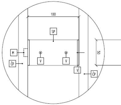
DET. 2 SPOJOVACÍ PRVKOK - PRIVARENÉ K PLECHU, DO DREVA VRUT
