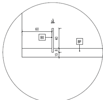
DET. 1 ZARÁŽKA VSADENÁ DO SPODNEJ POLICE
