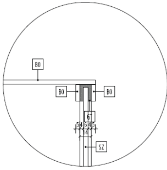
DET. 3 DRÁŽKA S GUMOVÝM TESNENÍM NA KOTVENÉ SKLENÉHO ZÁKLÖPU
