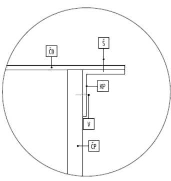
DET.1 KOTVIACI PRVKOV - PŘIVARENÉ K PLECHU, DO DŘEVA VRTUS
