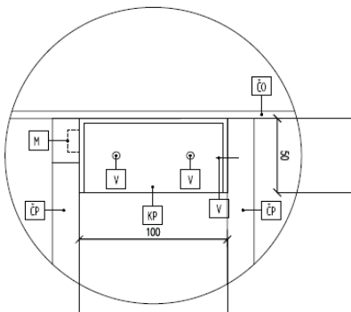
DET. 1 KOTVACÍ PRVKOV - PRIVÁRENÉ K PLECHU, DO DŘEVA VRUT
