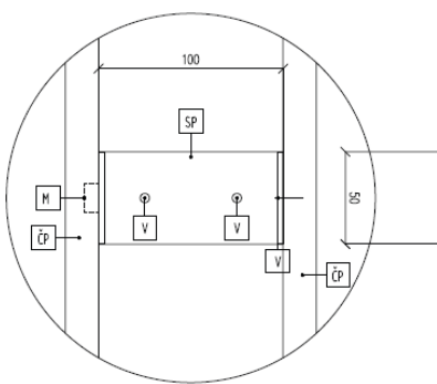
DET. 2 SPOJOVACÍ PRVKOV - PRIVÁRENÉ K PLECHU, DO DŘEVA VRUT
