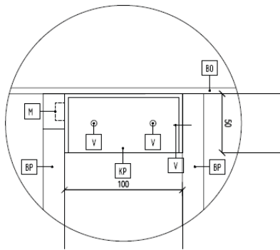
DET. 1 KOTVIACI PRVOK - PRIVARENÉ K PLECHU, DO DREVA VRUT
