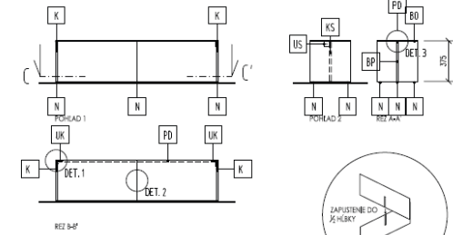
DET. 2 SCHÉMA ZAPŮSTENÝ SPOJ
