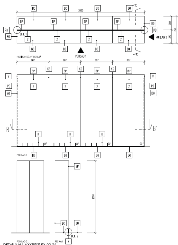
POHĽAD 2 DETAILY NA VÝKRESU EX-02-26
