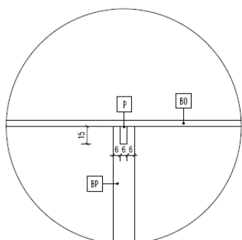
DET. 3 SPOJ - PERO-DRÁŽKA
