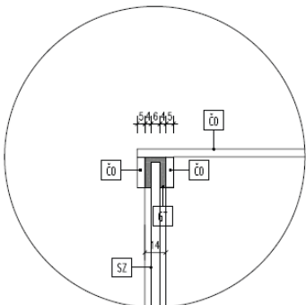
DET. 3 DRÁŽKA S GUMOVÝM TESNĚNÍM NA KOTVENÍ SKLENÉHO ZÁKLÖPU
