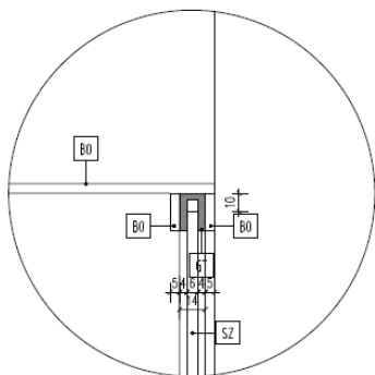
DET. 3 DRÁŽKA S GUMOVÝM TESNENÍM NA KOTVENÍ SKLENÉHO ZÁKLOPU
