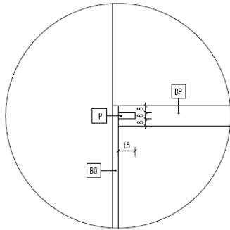
DET. 1 SPOJ - PERO-DRAŽKA
