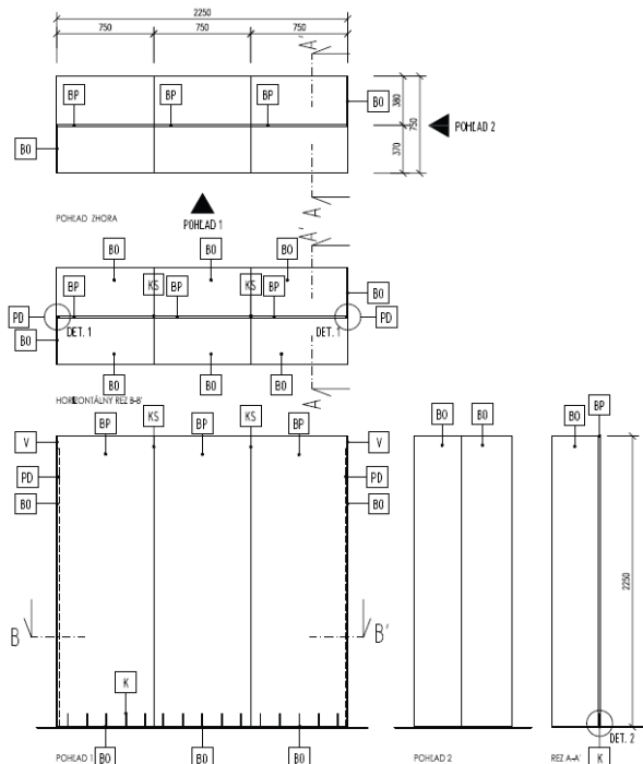
DETAILY NA VÝKRESE EX-02-02
