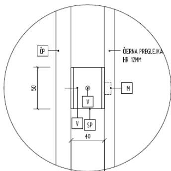
DET. 5 KOTVIACI PRVK - PRIVARENÉ K PLECHU, DO DREVA VRUT
