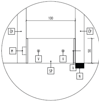
DET. 2 SPOJOVACÍ PRVOK - PRIVARENÉ K PLECHU, DO DŘEVA VRUT
