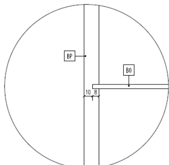
DET. 2 KOTVENIE POLICE DO BŔOHNICE
