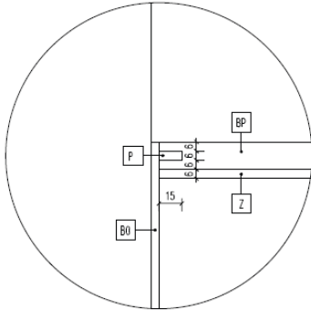
DET. 1 SPOJ - PERO-DRÁŽKA
