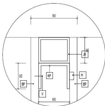
DET. 1 KOTVIACI PRVOK - PRIVARENÉ K PLECHU, DO DŘEVA VRUT
