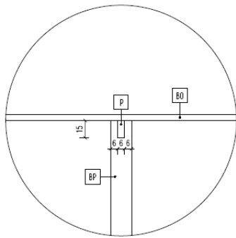
DET. 3 SPOJ - PERO-DŘÁŽKA
