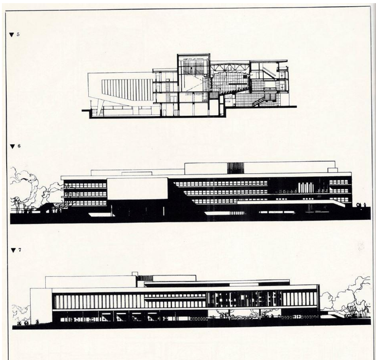
REZY A POHLÁDY pre znázornenie výškových úrovní strešnej roviny objektu.
