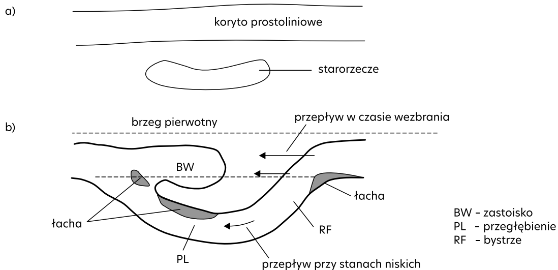
Rys. 60. Odtwarzanie zatok zastoiskowych na rzece Skerne, Darlington, Anglia [Krukowski 2006]
