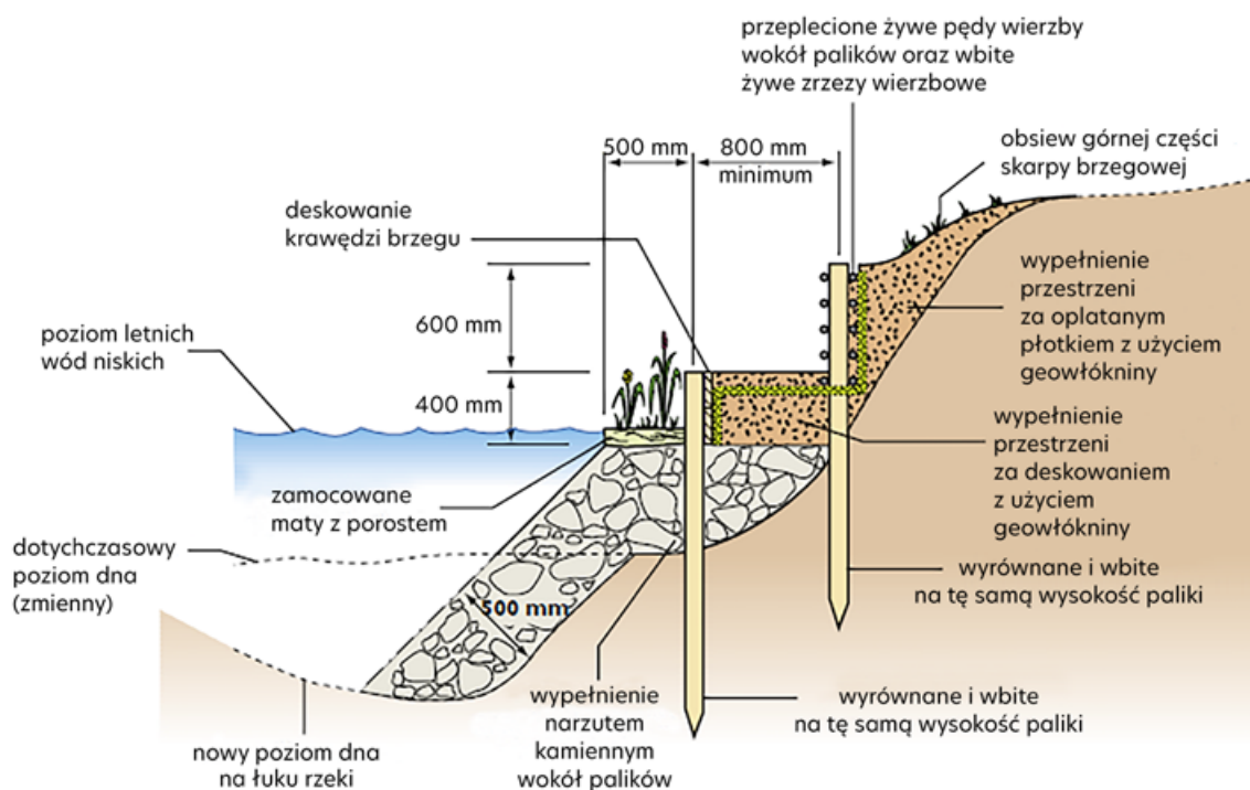
Rys. 73. Przekrój przez brzeg umocniony płotkiem plecionym [Krukowski 2006]
