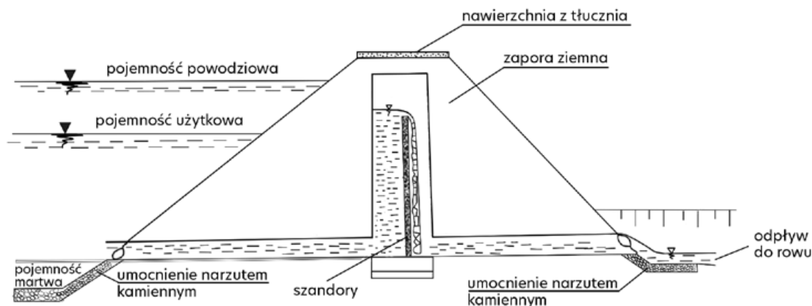
Rys. 20. Schemat zapory czołowej zbiornika ze studnią piętrząco-upustową (opracowano na podstawie: Biuro Projektowo-Wykonawcze „Hydrotechnika”)
