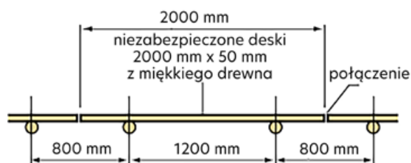
Rys. 74. Schemat deskowania krawędzi brzegu [Krukowski 2006]
