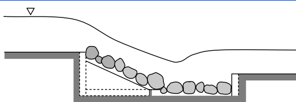
Rys. 97. Przebudowa stopni betonowych – bystrze z kamieni ułożonych na płycie dennej starego progu [Żelazo i Popek 2014]
