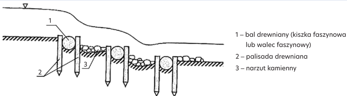
Rys. 45. Kaskada niskich progów drewnianych lub drewniano-faszynowych stabilizujących profil podłużny dna [Żelazo i Popka 2014]
