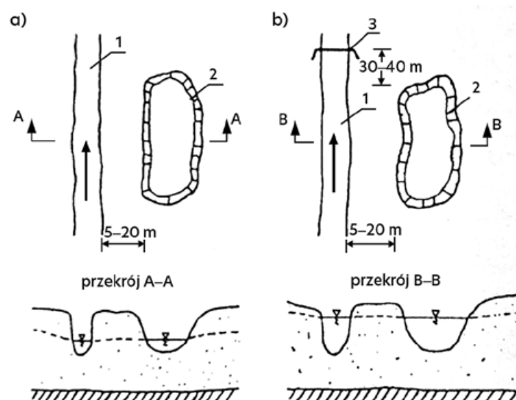
Rys. 13. Zbiornik zasilany infiltracyjnie z ciekłu: a) przy cieku naturalnym, b) przy cieku spiętrzymym [Mioduszeński 2014]
