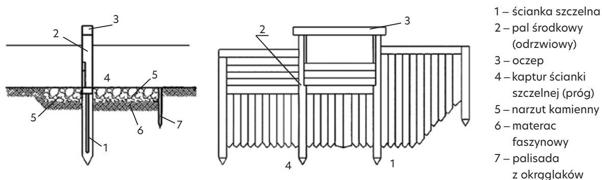
Rys. 26. Zastawka stosowana do małych piętrzeń [Biedroń 2018, na podstawie: Żbikowski 1969]
