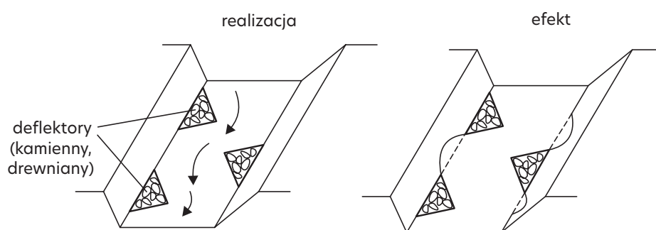
Rys. 53. Schemat naprzemienego rozmieszczania deflektorów/ostrog z materiałów naturalnych (rys. L. Książek)
