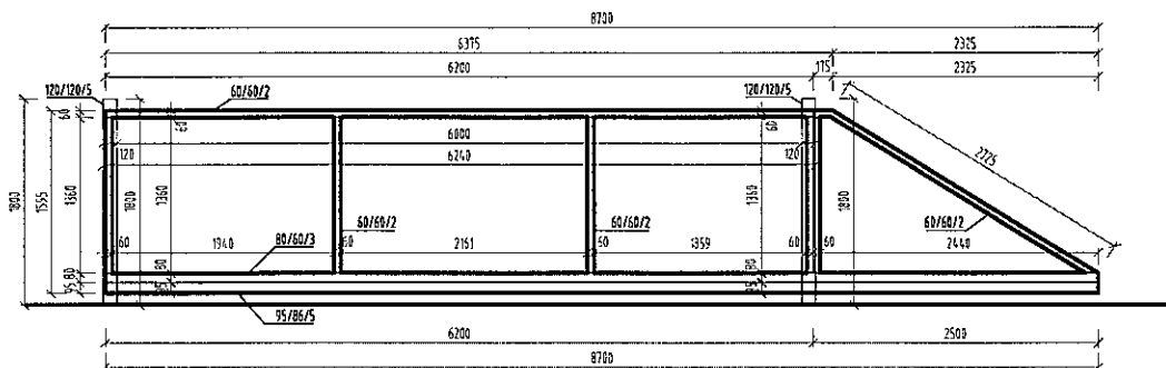
POHĽAD, NOSNÁ KONŠTRUKCIA BRÁNY M1:50
