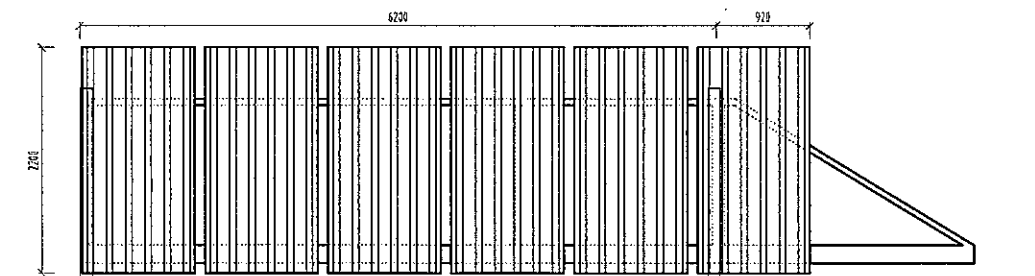
POHĽAD, VÝPLŇ BRÁNY M1:50
