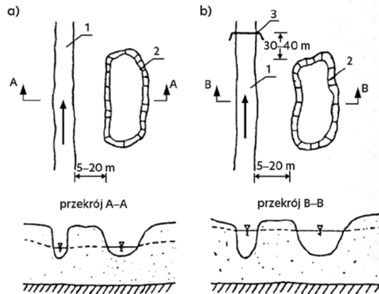
Rys. 13. Zbiornik zasilany infiltracyjnie z cieką: a) przy cieku naturalnym, b) przy cieku spiętrzoneym [Mioduszewski 2014]
