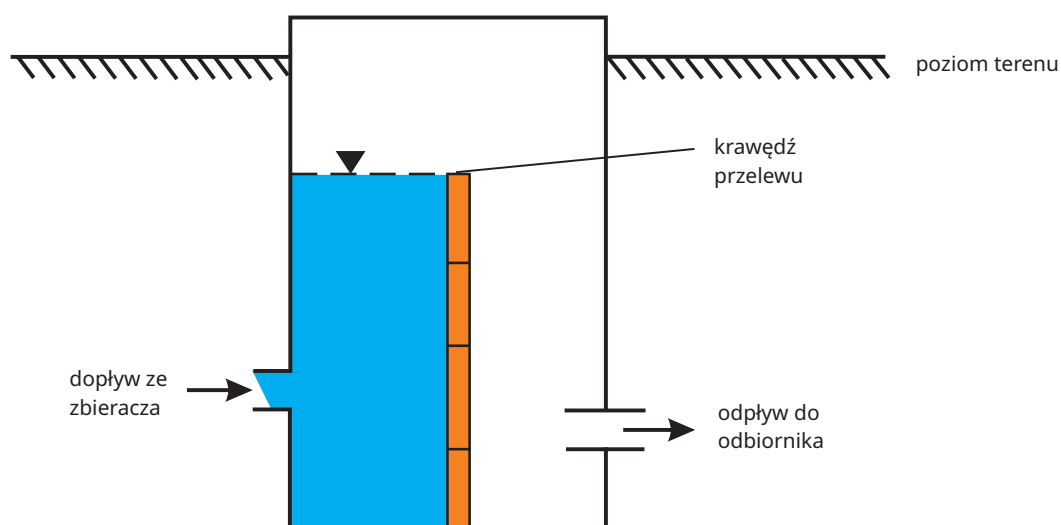
Rys. 50. Studnia piętrząca na zbieraczach przed wylotem [opracowano na podstawie: Mioduszewski [2003]
