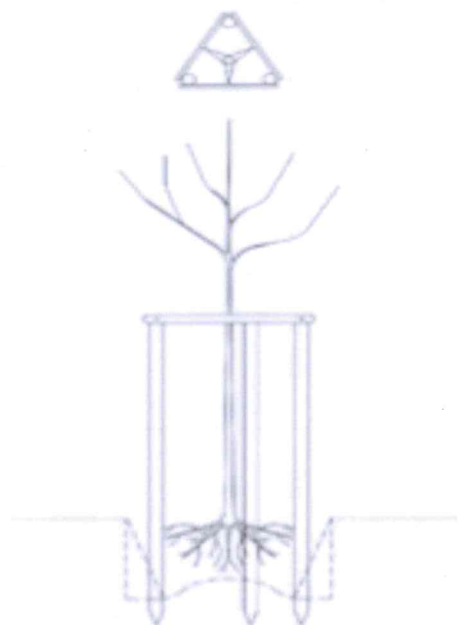
Obr. 1 - Nadzemné kotvenie stromov. Koly sa usadia do vykopanej jamy a umiestnia sa minimálne v hĺbke 200 mm do kompaktného (prírodného) terénu. Vrchol kolov môže siahať maximálne 100 mm pod korunu. Koly sa vzájomne priečne stabilizujú (Zdroj: Slovenská poľnohospodárska univerzita v Nitre: Arboristický štandard 4., Výsadba stromov a krov)
