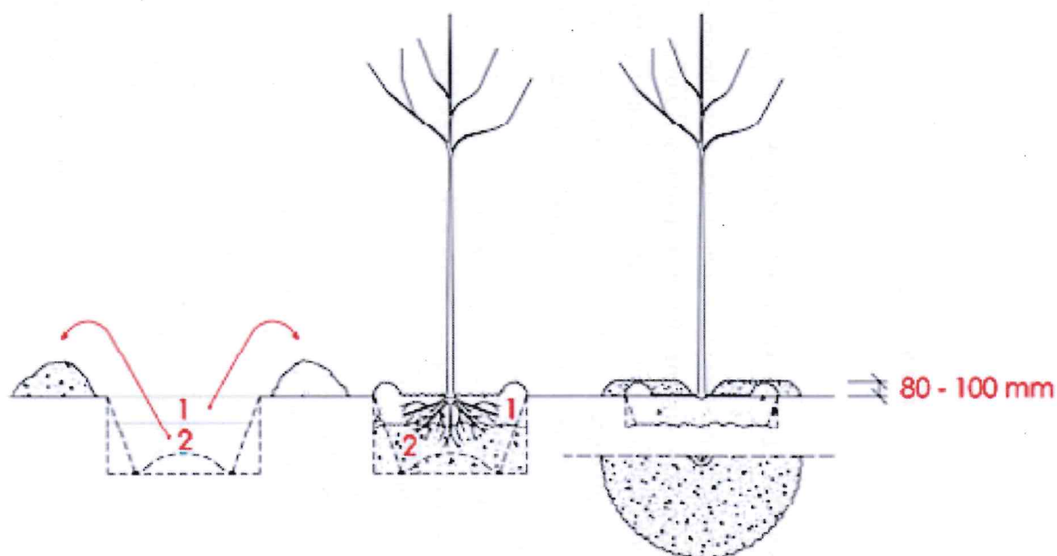
Obr. 2 - Spôsob výsadby a vytvorenia zavlažovacej misy s výškou steny 80 – 100 mm na rovine; (Zdroj: Slovenská poľnohospodárska univerzita v Nitre: Arboristický štandard 4., Výsadba stromov a krov)
