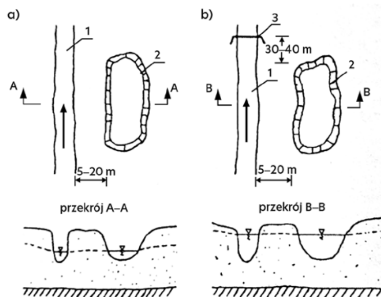
Rys. 13. Zbiornik zasilany infiltracyjnie z ciek: a) przy cieku naturalnym, b) przy cieku spiętrzym [Mioduszeński 2014]
