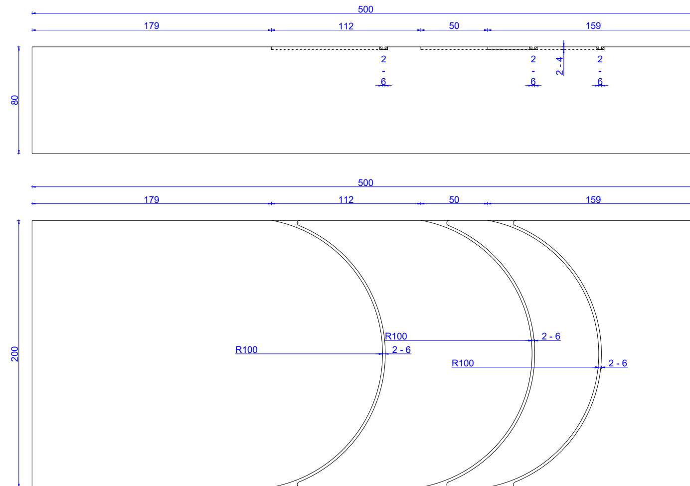
pôdorys
