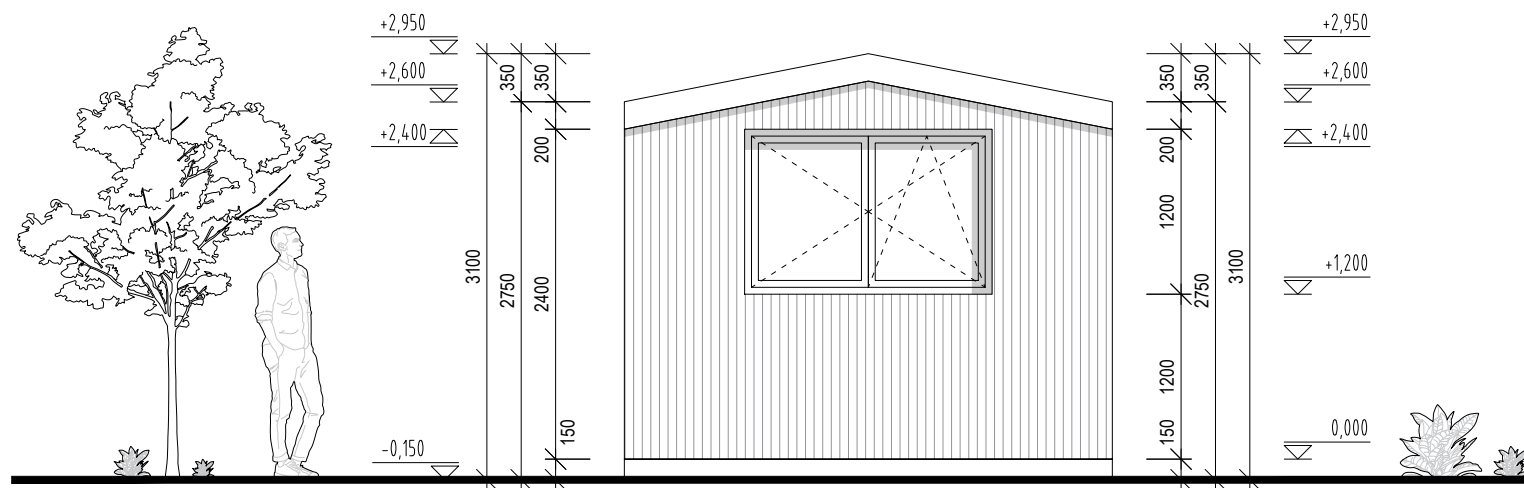
východný pohľad
