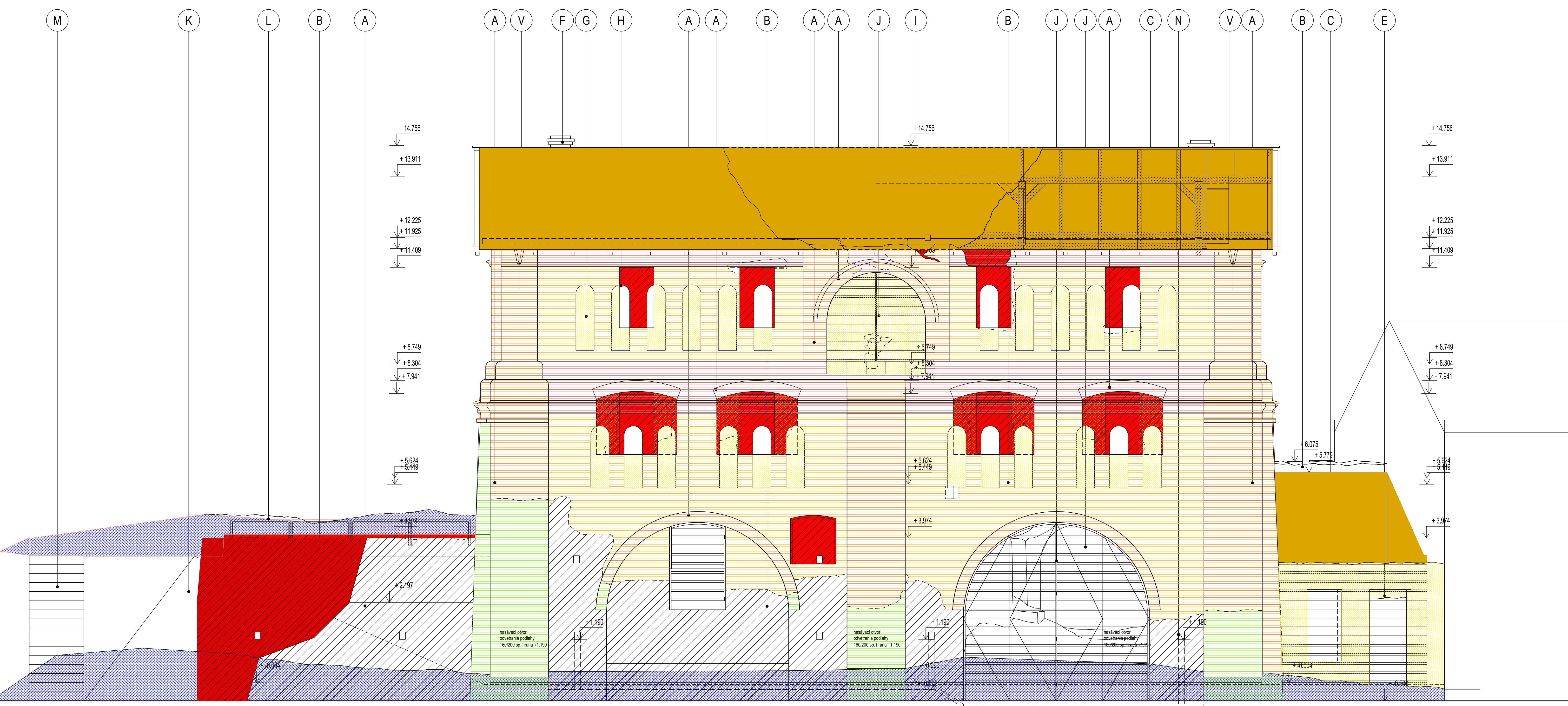
POHLAD JUŽNÝ - DELENIE DREVENNÝCH VÝPLŇÍ
