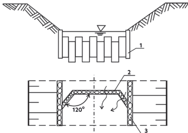
Rys. 41. Palisada w „ząbki” [Jędryka 2006]
