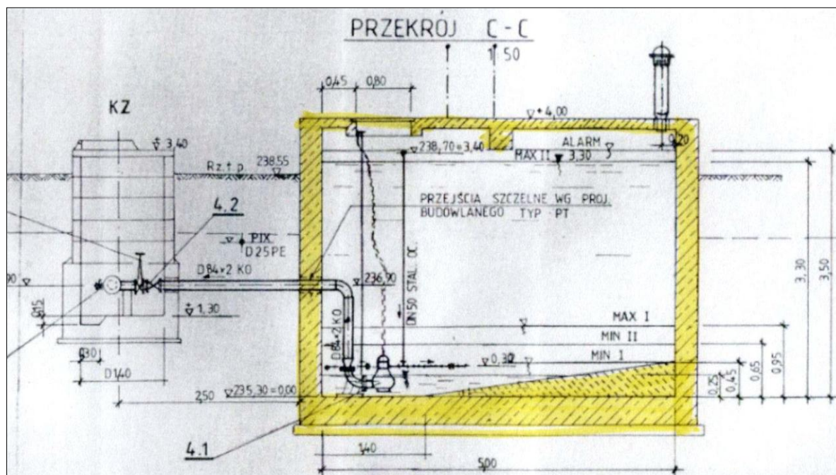
Rysunek 1.3.3-6 Zbiornik retencji i buforowania ścieków przed reaktorami SBR – rysunek poglądowy nr 3
