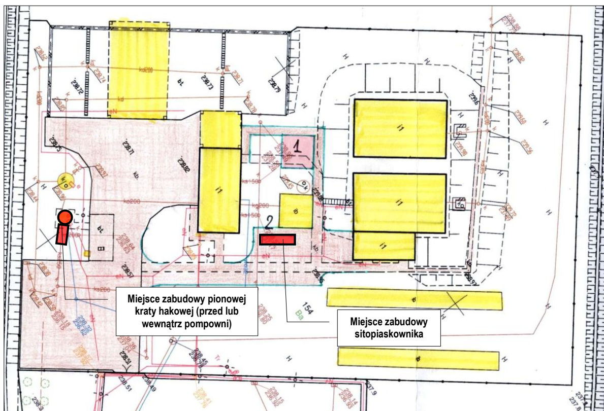
Rysunek 1.3.3-1 Poglądowa lokalizacja pionowej kraty hakowej i sitopiaskownika
