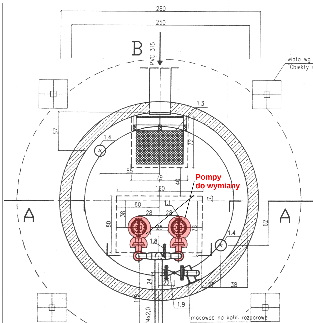
Rysunek 1.3.3-2 Usytuowanie przeznaczonych do wymiany, istniejących pomp zatapialnych w pompowni głównej
