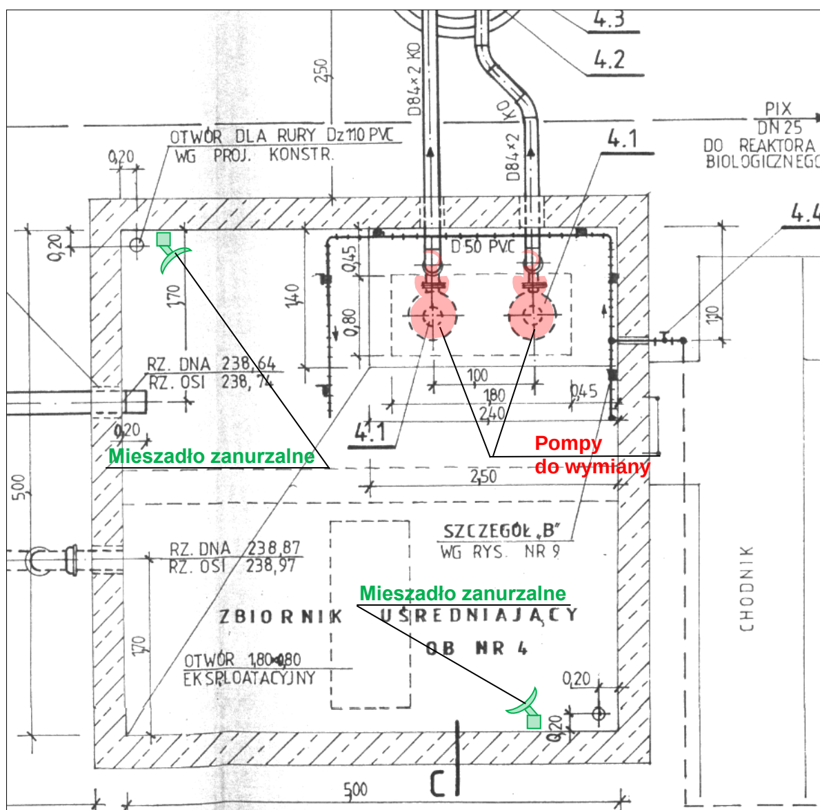
Rysunek 1.3.3-7 Poglądowe usytuowanie nowego mieszadła zanurzalnego w zbiorniku uśredniającym
