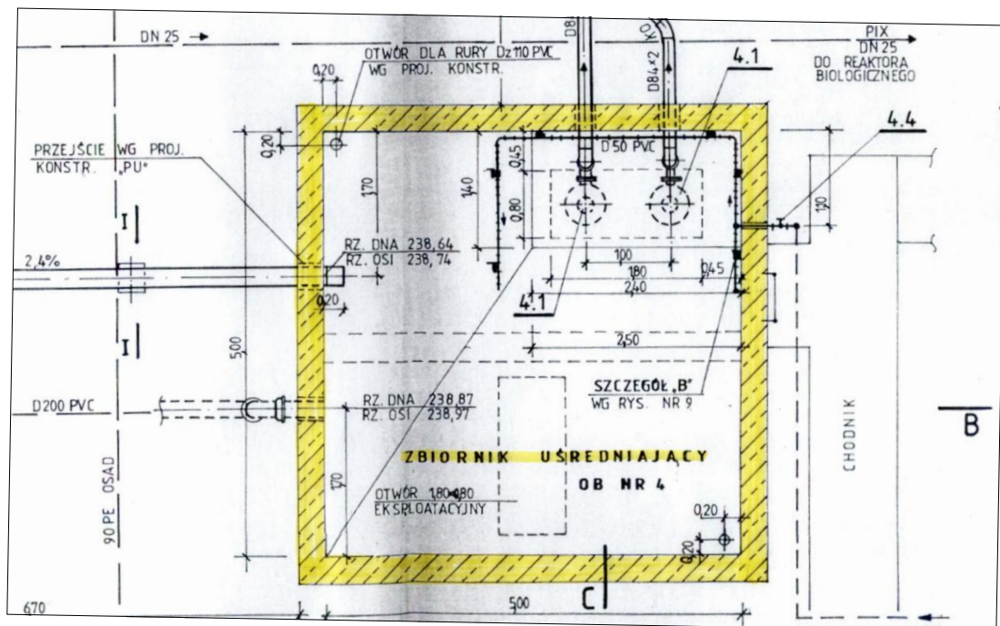
Rysunek 1.3.3-4 Zbiornik retencji i buforowania ścieków przed reaktorami SBR – rysunek poglądowy nr 1
