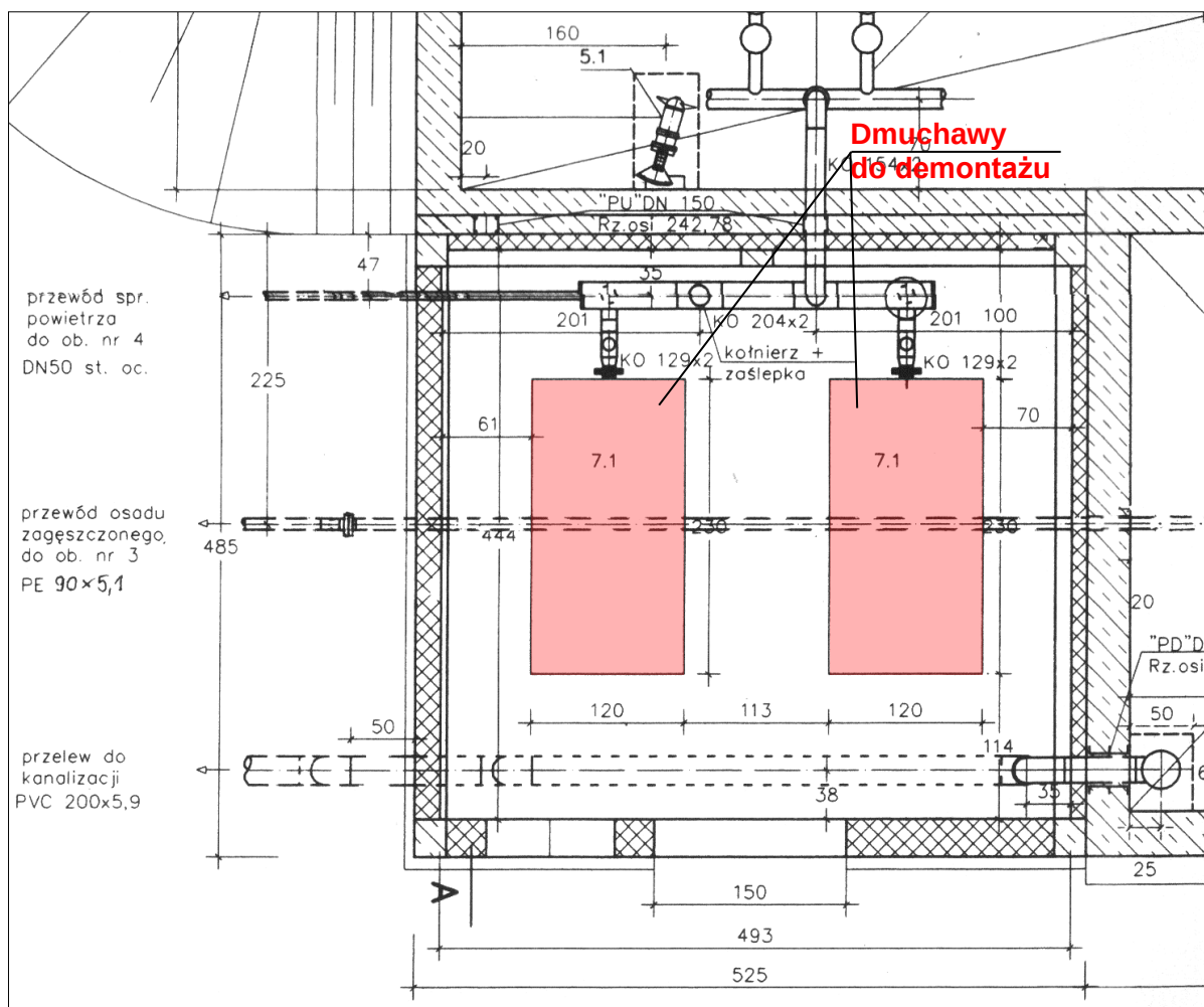
Rysunek 1.3.3-3 Rzut istniejącego pomieszczenia dmuchaw
