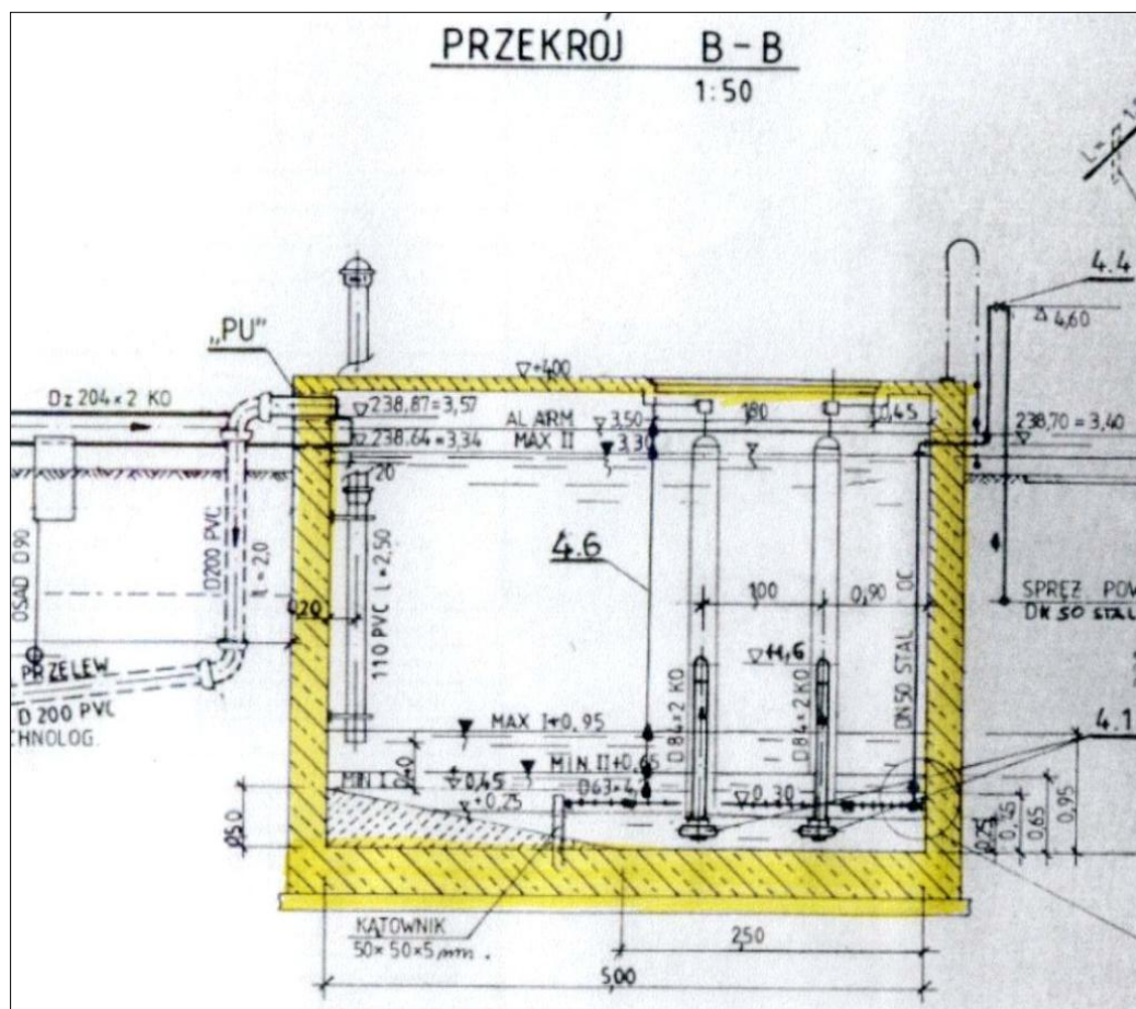
Rysunek 1.3.3-5 Zbiornik retencji i buforowania ścieków przed reaktorami SBR – rysunek poglądowy nr 2
