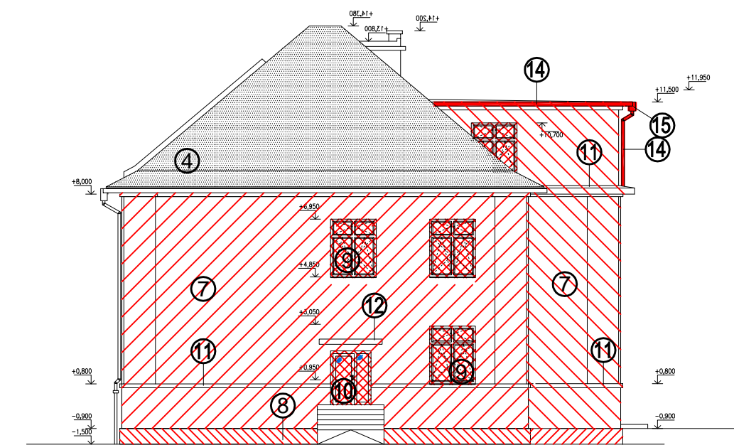
JUHOZÁPADNÝ POHLAD
