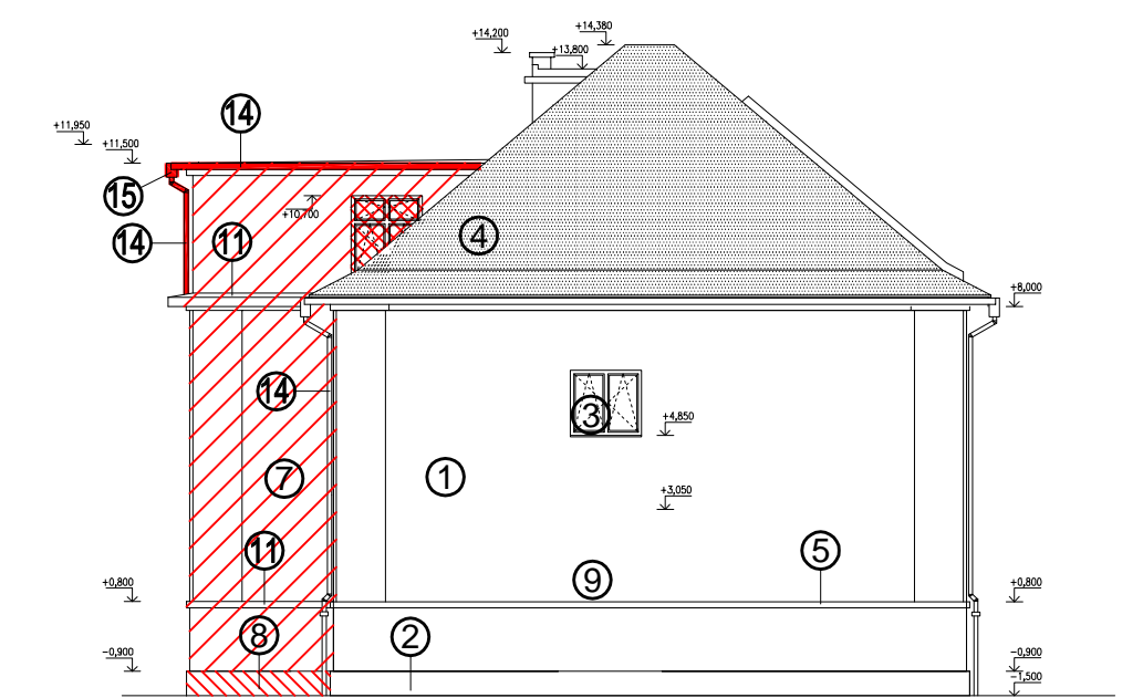
JUHOVÝCHODNÝ POHLAD
