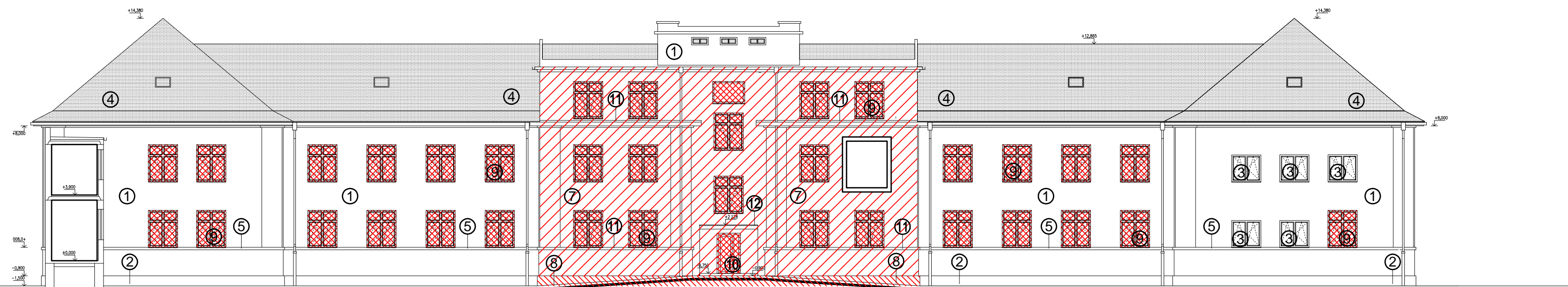
SEVEROZÁPADNÝ POHLAD
