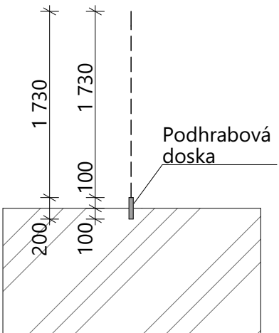
Rez - pletivo
