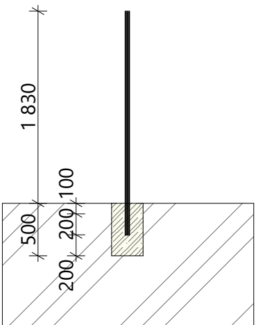
Rez - stĺpik
