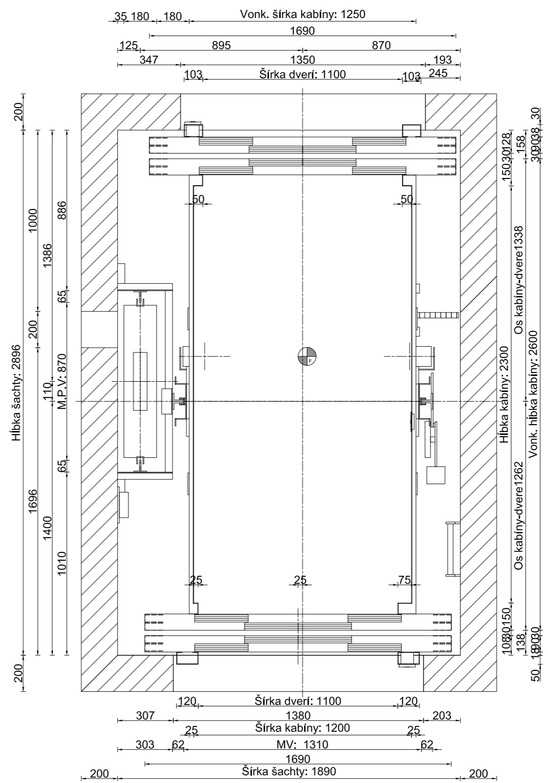
Pôdorys šachty:
